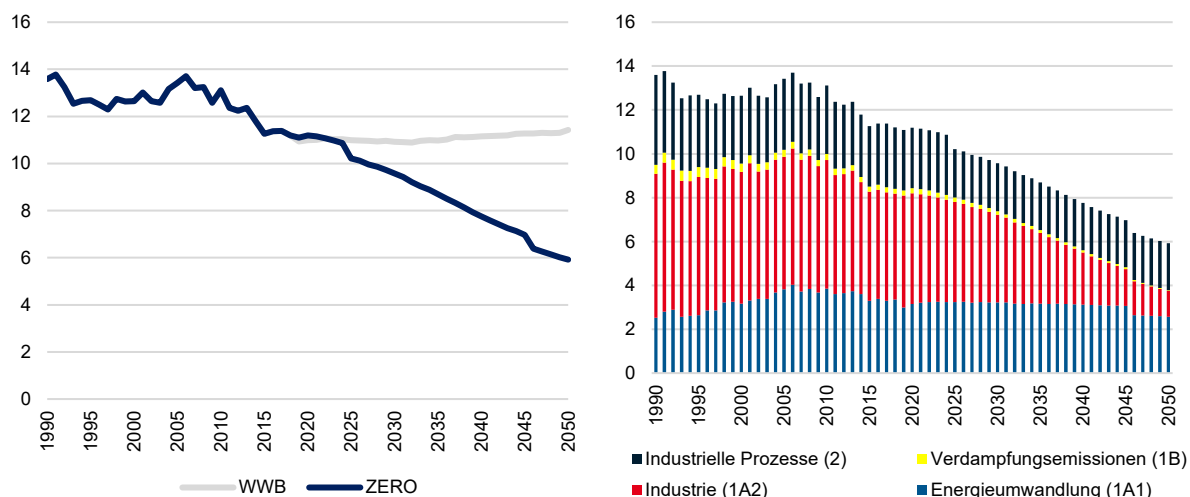
Abbildung 16: Entwicklung der Treibhausgasemissionen im Sektor Industrie insgesamt (links) und nach Kategorien (rechts, nur Szenario ZERO Basis) in Mt CO 2 eq gemäss EP2050+, jeweils ohne CCS und NET. Quelle: Prognos/TEP Energy/Infras/Ecoplan 2020.
